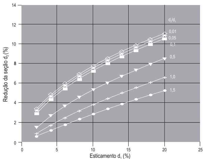
Diagrama 8.3 Redução da seção em função do aumento do diâmetro interno ( d_2/d_1 )
