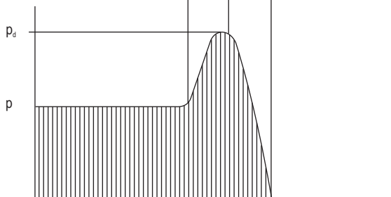
Ilust. 6.9 Efeito de vedação automático das gaxetas elásticas
