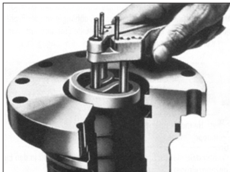
Ilust. 6.23 Ferramenta de montagem para gaxetas de haste
