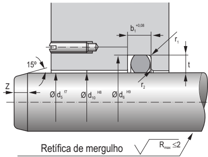
Dimensões do canal retangular para anéis O’rings em caso de movimentos rotativos.
