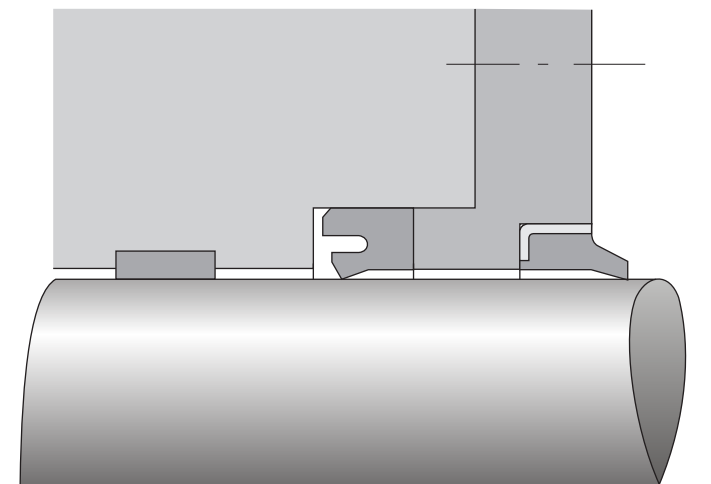
Recomendação de montagem II
