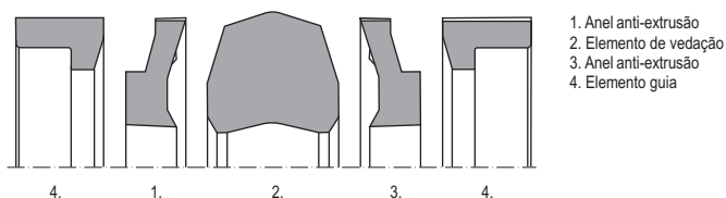
Ilust. 4.36 Montagem de gaxeta compacta de êmbolo L43
