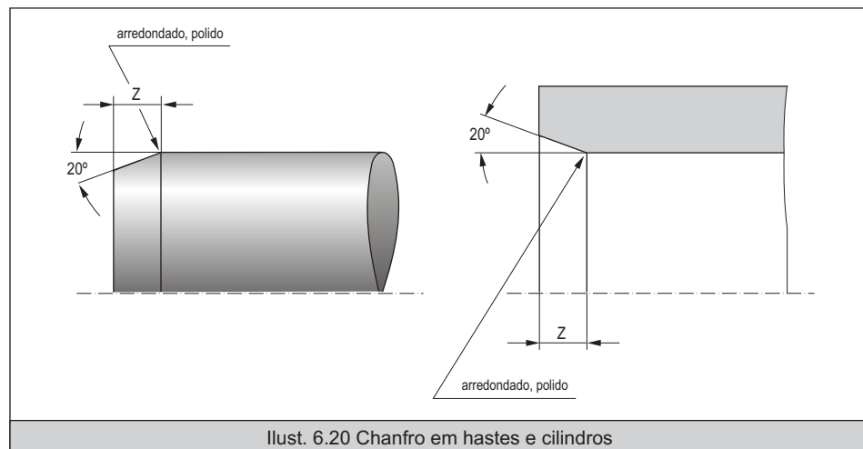
Ilust. 6.20 Chanfro em hastes e cilindros
