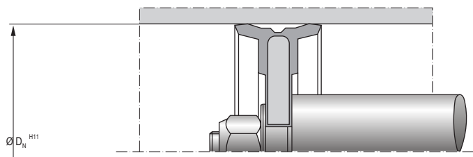
Ilust 6.18 Ajustes e tolerâncias para gaxetas e elemento guia
