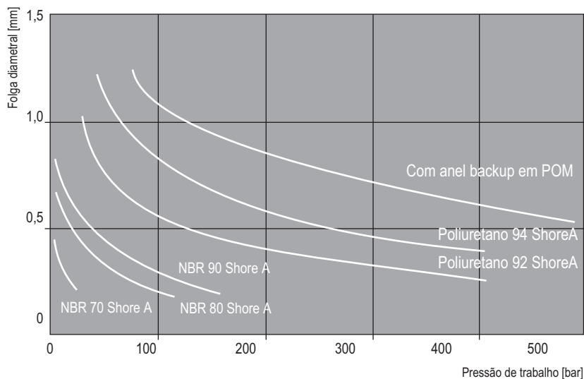
Ilust. 4.16 Folga diametral em função da pressão
