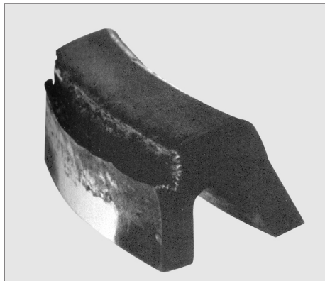
Ilust. 4.17 Extrusão na gaxeta U
