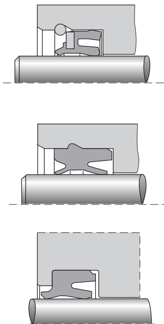
Ilust. 6.27 Montagem de gaxeta-raspador
