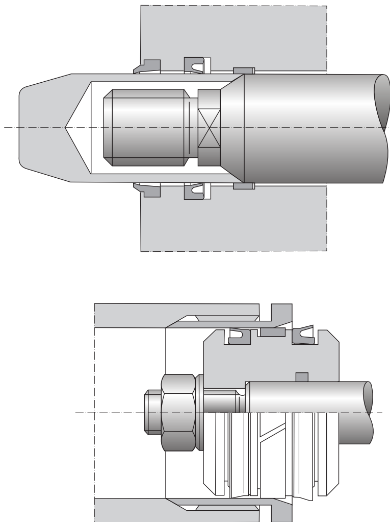
Ilust. 6.21 Recobrimento de roscas durante a montagem de gaxetas
