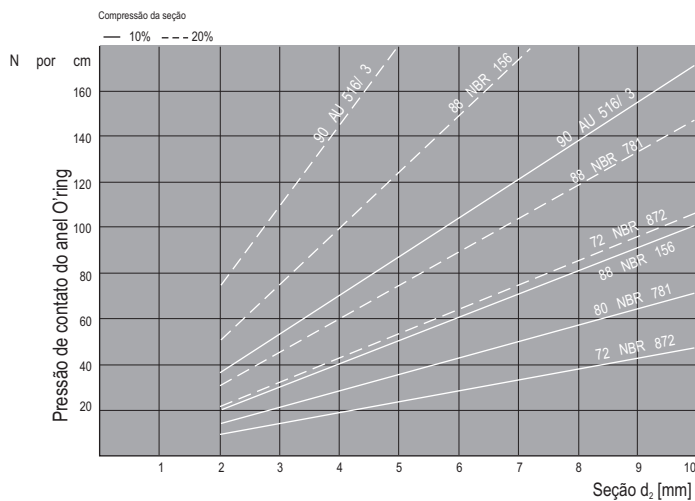
Diagrama 8.4 Pressão de contato em caso de deformações de 10 e 20%
