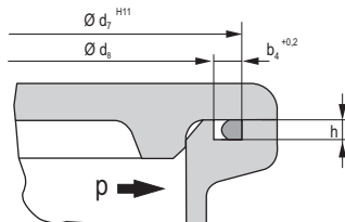
Pressão de dentro para fora
