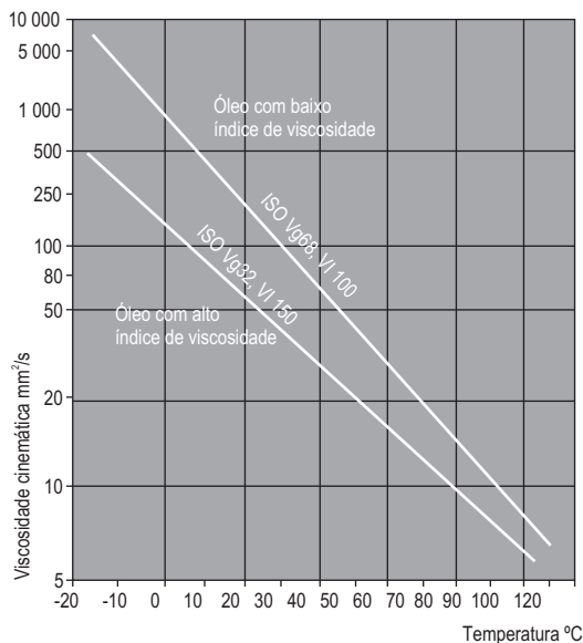
Ilust 4.15 Comportamento, viscosidade - temperatura de vários óleos hidráulicos
