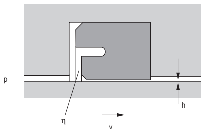
Ilust. 4.9 Aumento da pressão e formação do filme lubrificante
