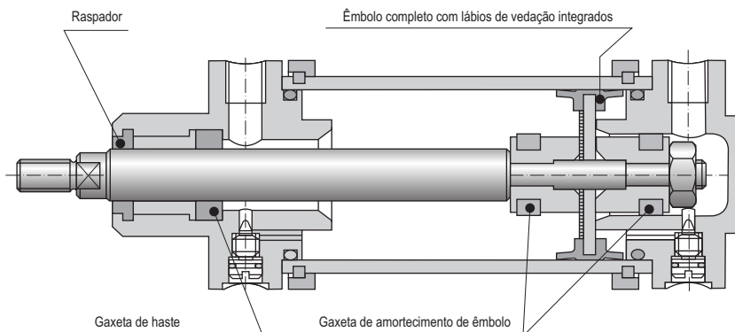
Ilust. 6.3 Cilindro pneumático II
