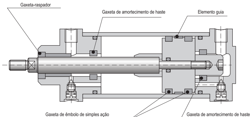
Ilust. 6.4 Cilindro Pneumático III
