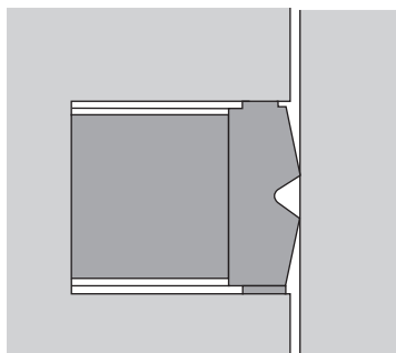
Ilust. 4.3 Gaxeta de êmbolo
