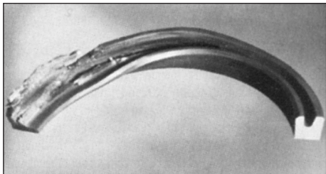
Ilust 4.12 Gaxeta U destruída por aumento da pressão hidrodinâmica
