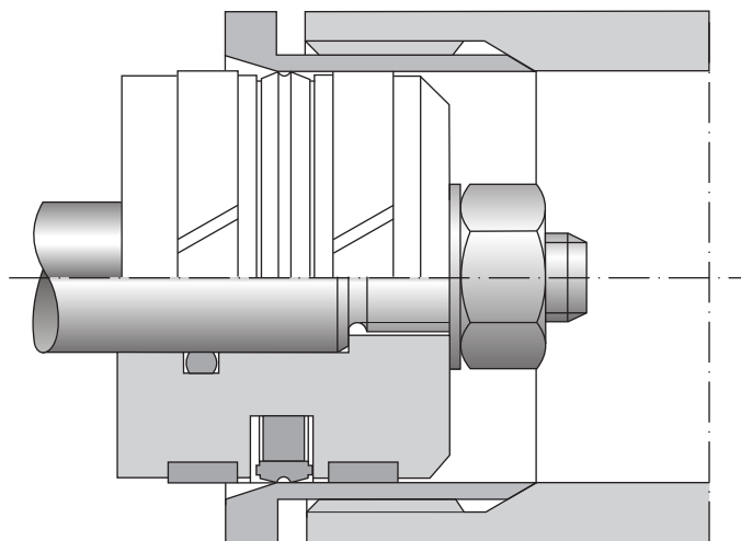
Ilust. 4.22 Recobrimento de roscas durante a montagem de gaxetas
