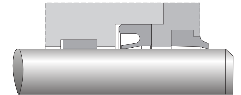
Ilust. 6.22 Tipos de montagem para gaxetas de haste
