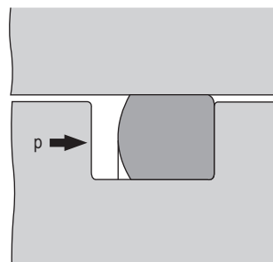
Deformado sob pressão
