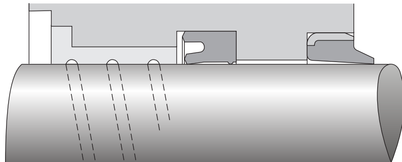
Canais de alívio de pressão em guias metálicas
