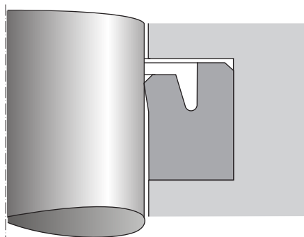
Ilust. 4.2 Gaxeta de haste
