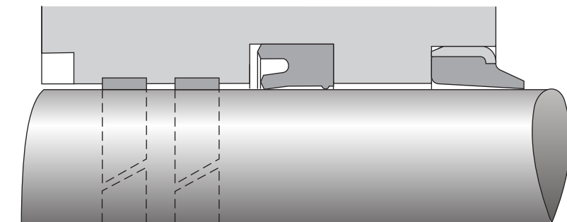
Folga produzida pelas guias plásticas
