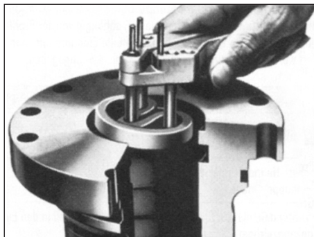
Ilust. 4.24 Ferramenta de montagem para gaxetas de haste
