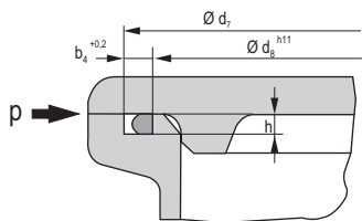
Pressão de fora para dentro
