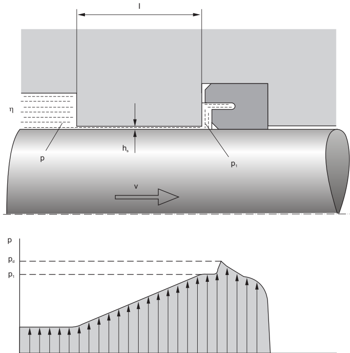
Ilust 4.11 Fluxo de arraste hidrodinâmico
