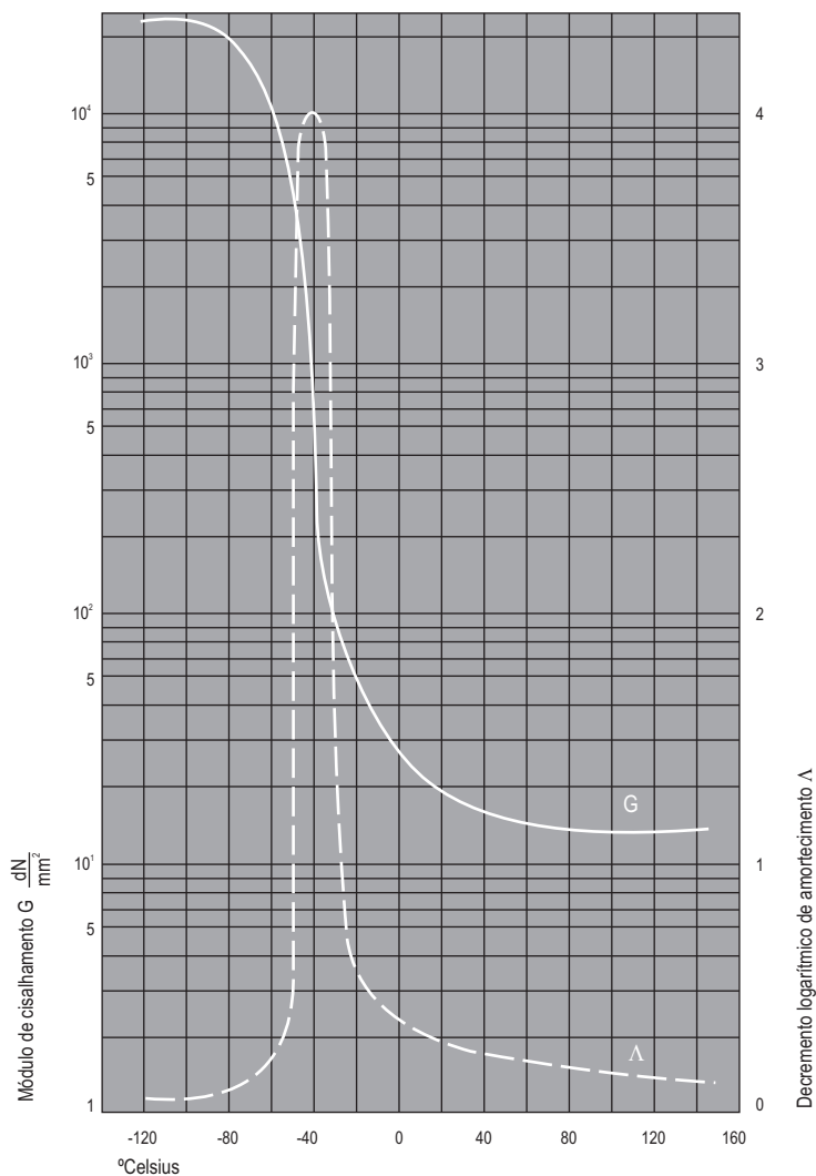
Ilust. 4.14 Diagrama: teste de vibração torcional conforme DIN 53445; módulo de cisalhamento dinâmico G e decremento logarítmico \Delta de material Simirit a base de CR
