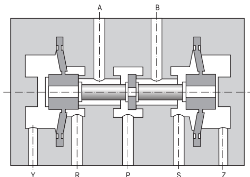
Ilust. 6.8 Válvula distribuidora 5/2
