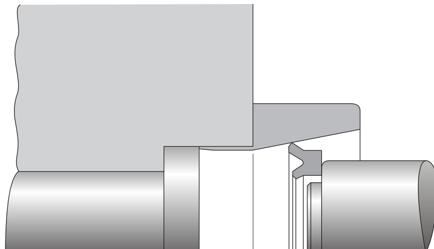
Ilust. 4.27 Montagem de gaxtas de haste em alojamentos bi-partidos
