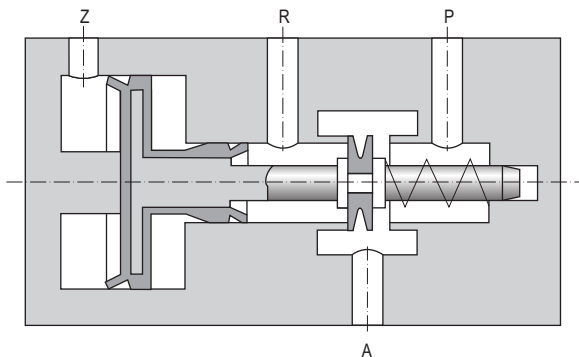
Ilust. 6.7 Válvula distribuidora 3/2
