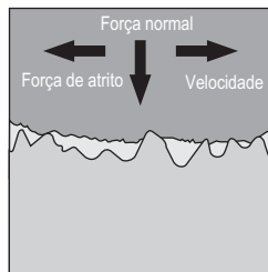
Atrito misto (M)
