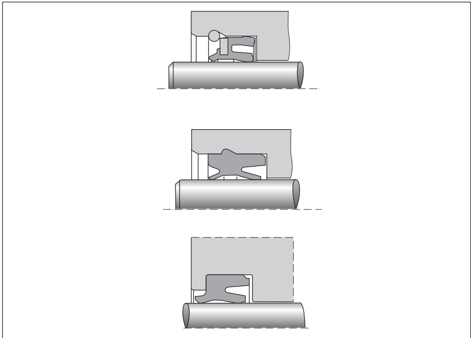
Ilust. 6.27 Montagem de gaxeta-raspador
