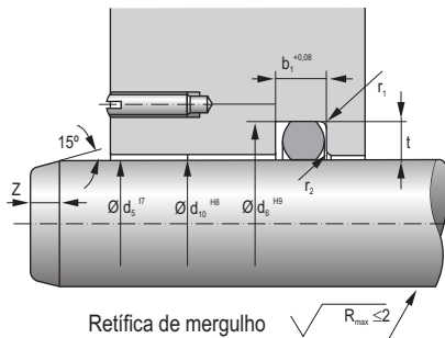
Dimensões do canal retangular para anéis O’rings em caso de movimentos rotativos.
