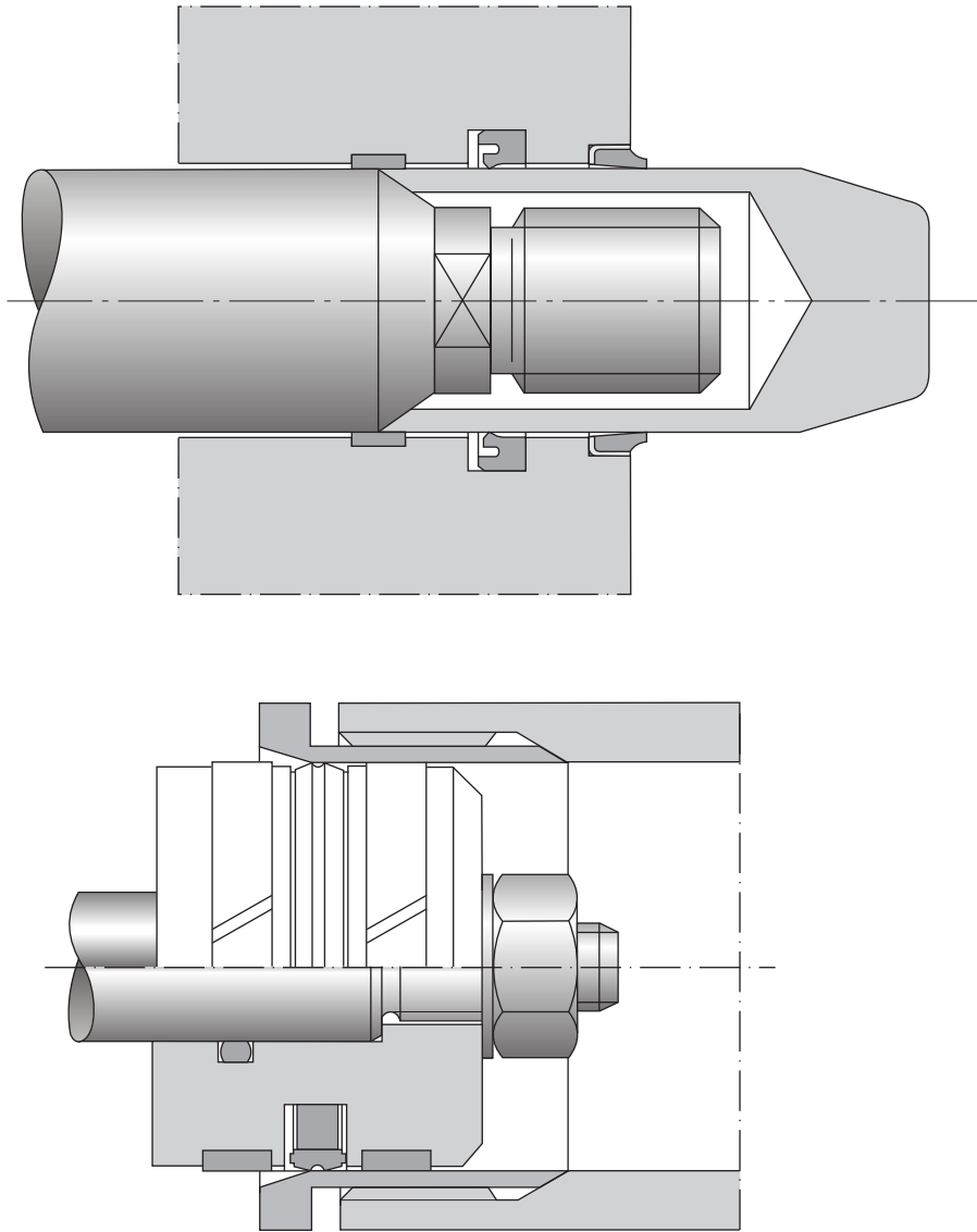
Ilust. 4.22 Recobrimento de roscas durante a montagem de gaxetas
