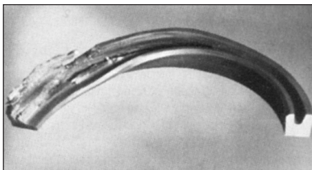
Ilust 4.12 Gaxeta U destruída por aumento da pressão hidrodinâmica
