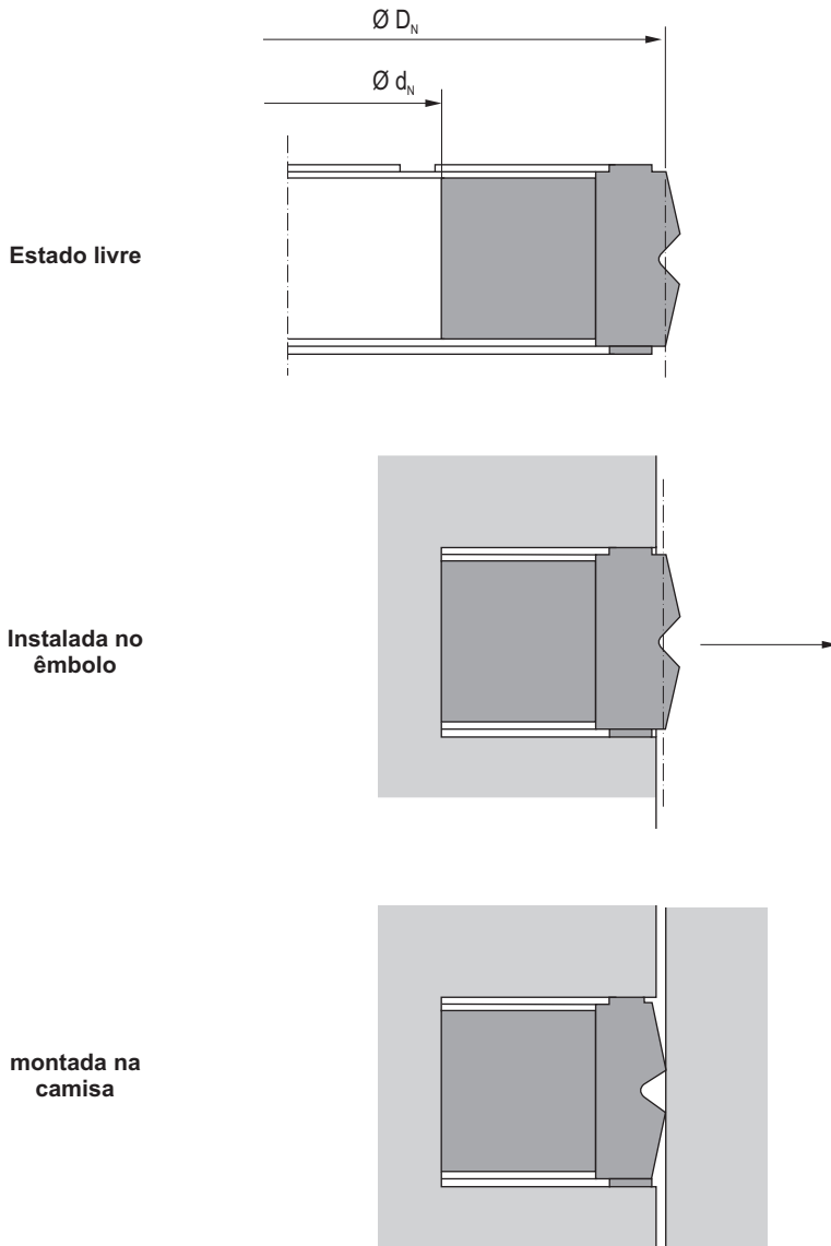
Ilust. 4.3 Gaxeta de êmbolo
