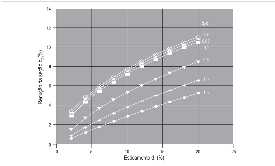
Diagrama 8.3 Redução da seção em função do aumento do diâmetro interno ( d_2/d_1 )
