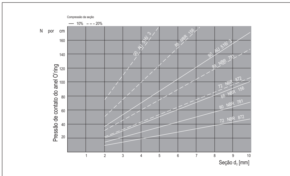
Diagrama 8.4 Pressão de contato em caso de deformações de 10 e 20%
