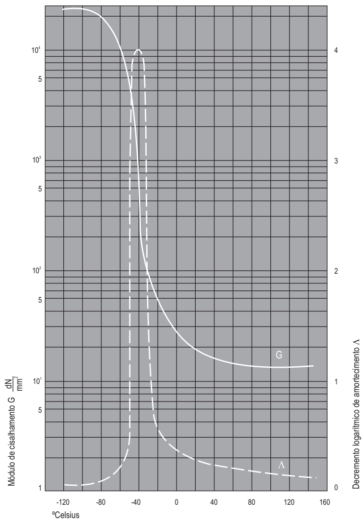
Ilust. 4.14 Diagrama: teste de vibração torsional conforme DIN 53445; módulo de cisalhamento dinâmico G e decremento logarítmico \Delta de material Simirit a base de CR
